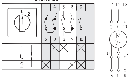
3-полюсные, возврат в положение «0» Схема 26
