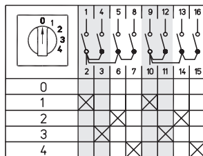
2-полюсные, 4 позиции Схема 125
