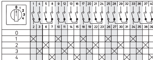
6-полюсные, 2 позиции
