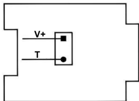
4...20 мА
