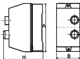
Пускатель номинальный ток 10А, 16А. Степень защиты - IP40, IP54
