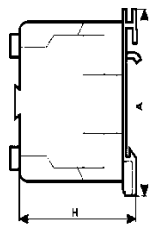
Пускатель реверсивный номинальный ток 25А, 32А
