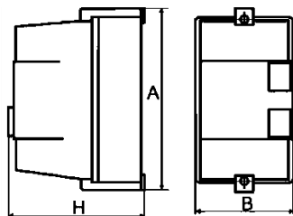
Пускатель номинальный ток 25А, 32А. Степень защиты - IP40, IP54
