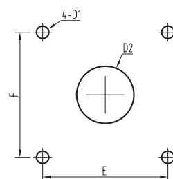
Монтажные размеры
