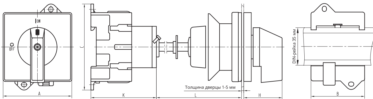
Монтажные размеры
