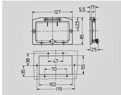
Чертеж 6 МВ 4
