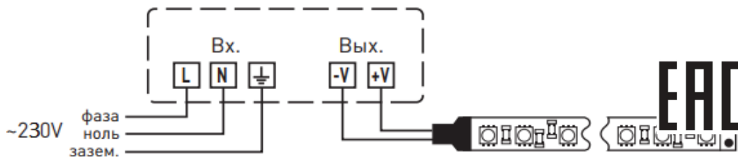
Рисунок 1 – Схема подключения
