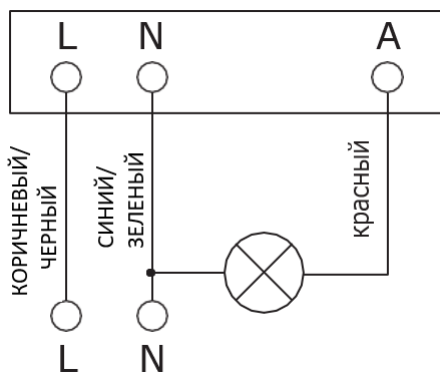
Рисунок 4. Схема подключения датчика MD 018 и MD 019
