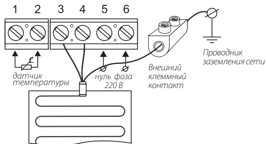
Рисунок 2. Схема подключения мата к сети (220 В)
