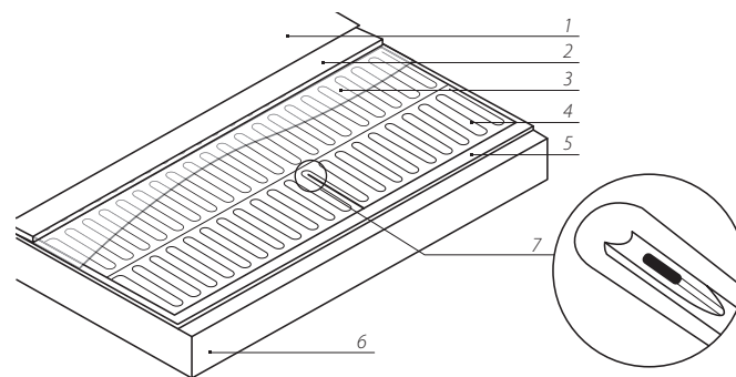
Рисунок 7. Конструкция элементов пола с использованием в качестве финального покрытия линолеума или ковролина
