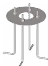
Комплект анкерных болтов АВ 178. Код заказа – 2407000020
