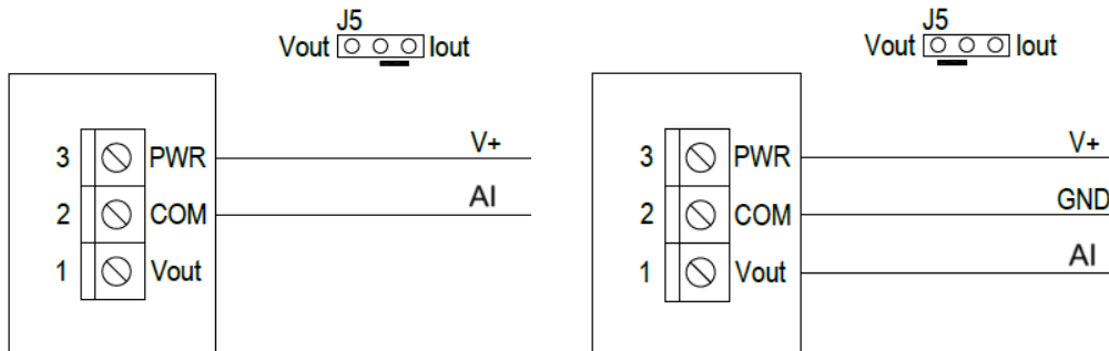
Подключение по двухпроводной схеме сигнала 4...200 мА к аналоговому входу контроллера
