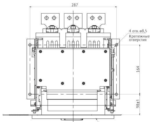
S1 выдвижного типа с установленной рамкой (вид сверху)
