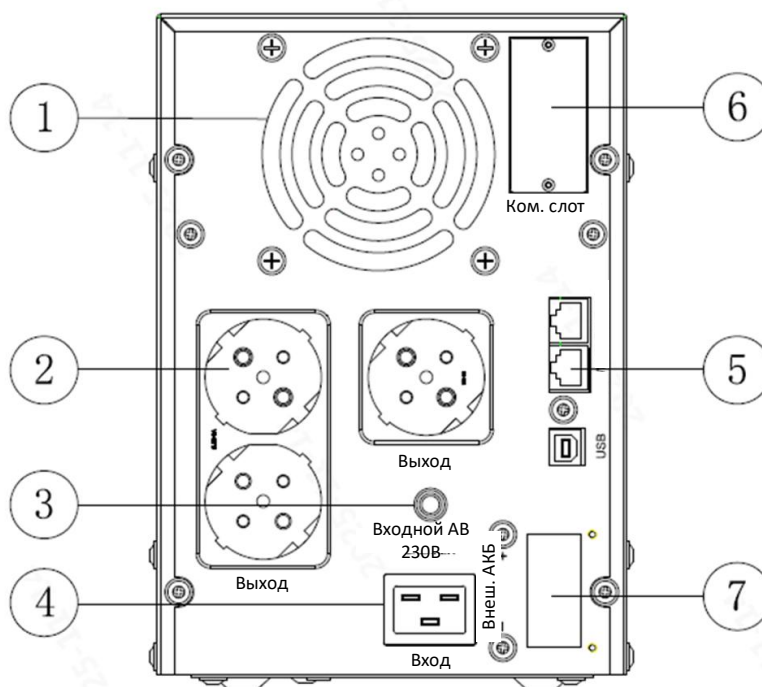
Рисунок 7-2. Вид сзади
