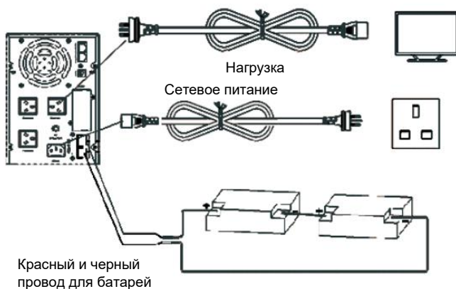
Рисунок 8-3. Подключение ИБП с внешней батареей 24В
