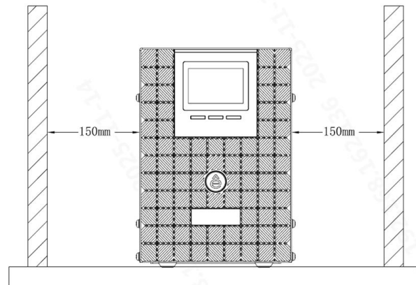
Рисунок 8-1. Рекомендации по установке
