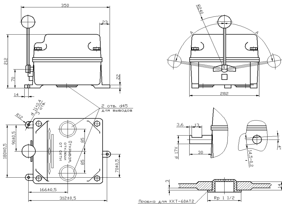
Рисунок. Габаритные и установочные размеры
