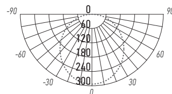
PPL 089/G OPAL 9W
