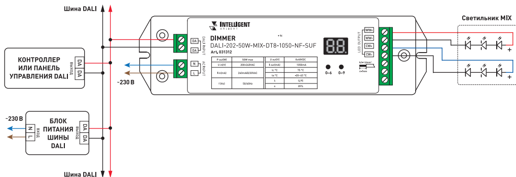
Рисунок 1. Пример схемы подключения диммера DALI-202-50W-MIX-DT8-1050-SUF
