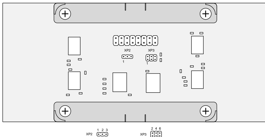
Рисунок 2 – Расположение перемычек XP2 и XP3
