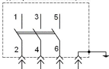
для трехполюсных ящиков
