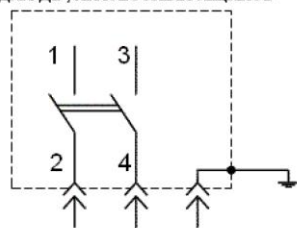
для двухполюсных ящиков
