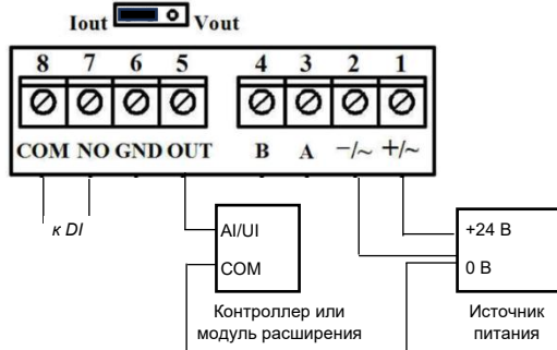
Схема подключения выходного сигнала 4...20 мА
