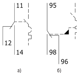
а) ВА47-МСК; б) ВА47-МССК.
