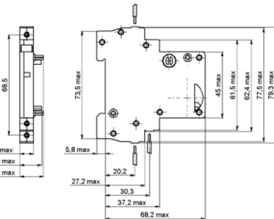
Рисунок 1 – Габаритные размеры МВК
