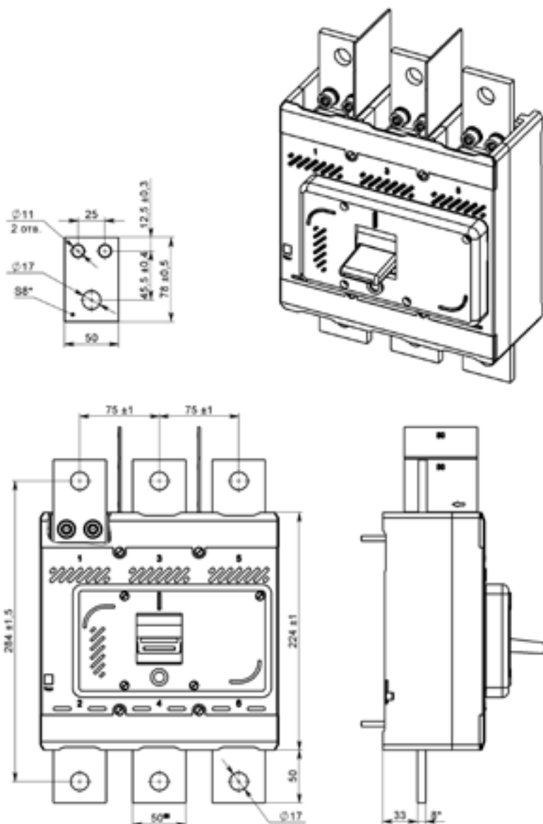
Рисунок 3а – Присоединение с переходной шиной
