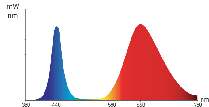
Спектрограмма излучения
