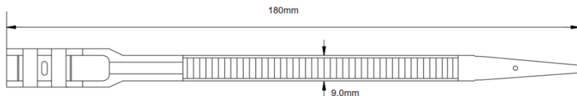
Рисунок 1 Кабельные стяжки 9.0 x 180 мм
