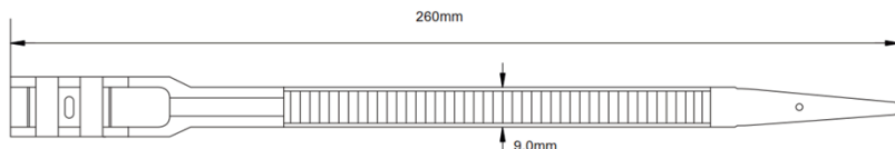
Рисунок 2 Кабельные стяжки 9.0 x 260 мм
