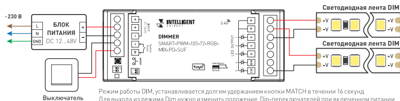
Рис. 1. Схемы подключения диммера SMART-PWM-105-72-RGB-MIX-PD-SUF
