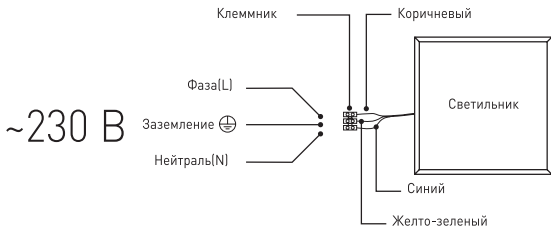
Рис.1. Схема подключения светильника к сети 230В.
