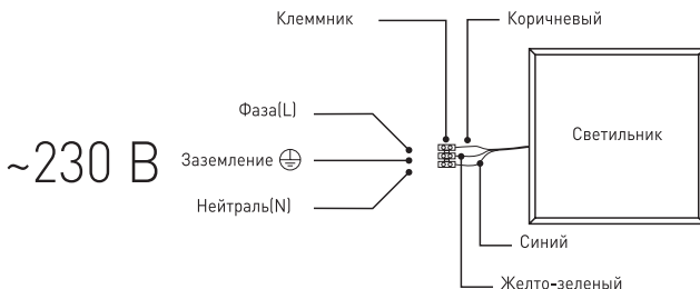
Сурет. 1. Шамды 230В желіге қосу схемасы.
