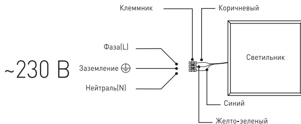
Բրիժ.1. Միացման սխեման lamp ցանցի 230V.
