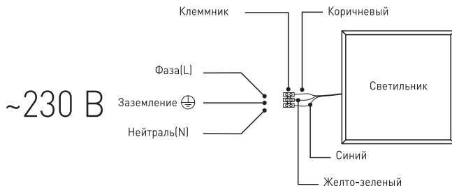
- Сүрөт.1. Кошулуу схемасы светильника тармагына 230В.
