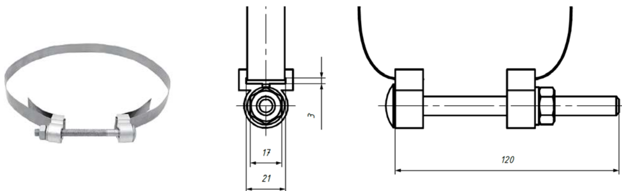
Рис. 1. Внешний вид крепежного хомута BF 207.
