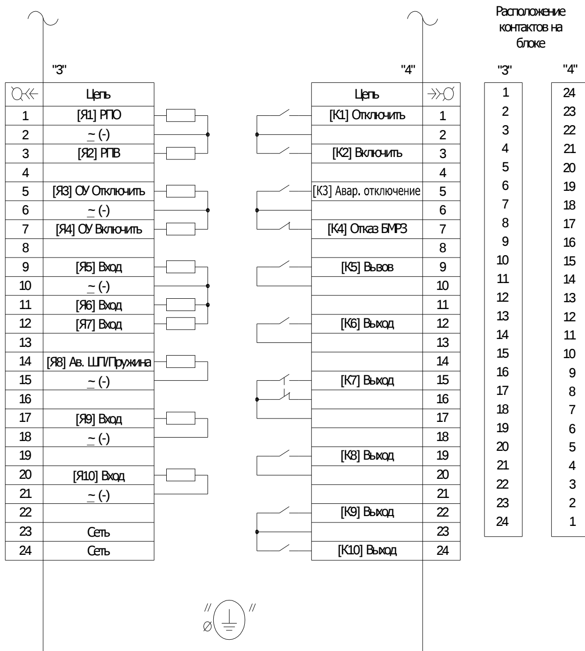
Рисунок А.3 - Схема электрическая подключения БФПО
