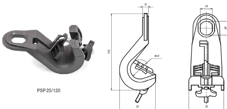
Рис. 1. Внешний вид поддерживающего зажима PSP 25/120.
