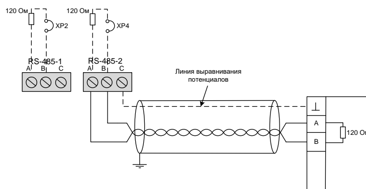
Рисунок 8 – Подключение интерфейса RS-485
