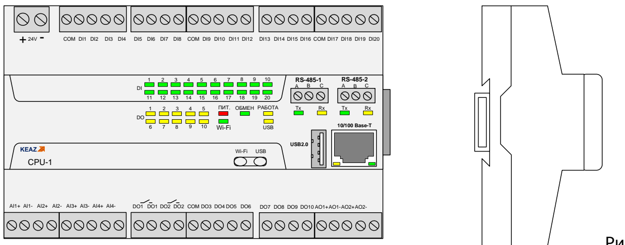
суюнок 1 – Внешний вид и размеры модуля
