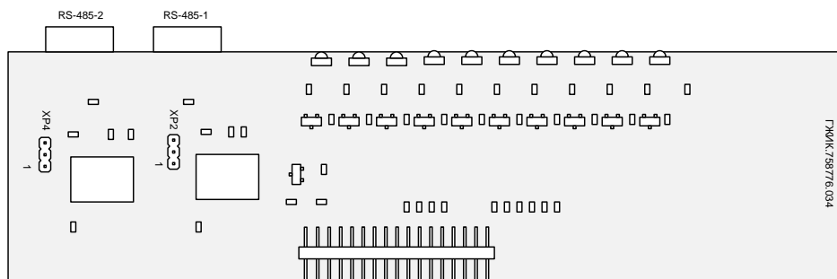
Рисунок 5 – Расположение перемычек XP2 и XP4
