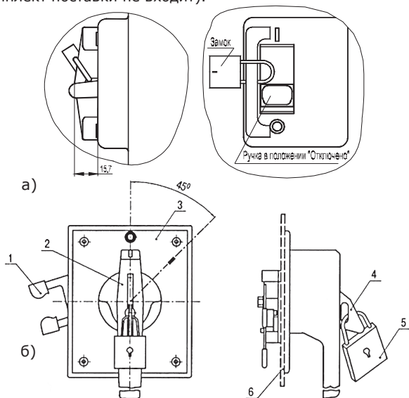
а) выключателей стационарного исполнения с ручным приводом, б) выключателей с ручным дистанционным приводом (1 - поводок, 2 - рукоятка, 3 - основание, 4 - пластина, 5 - замок, 6 - дверь распределительного устройства)
