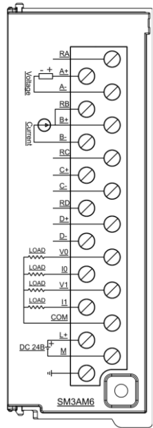
Расположение и назначение клемм
