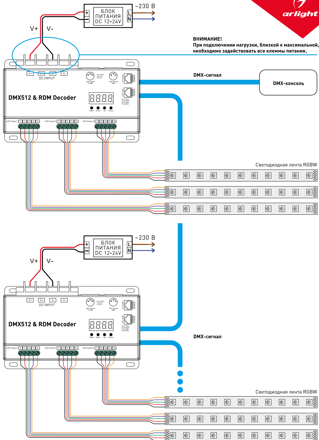
Рис. 2. Схема подключения декодера.
