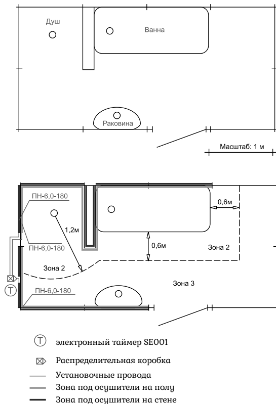
Рисунок 8. Определение размеров зон обогрева в случае установки осушителей в пол и прилегающую к полу часть стены (бордюр).
