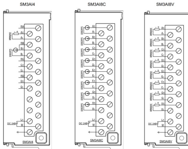
Расположение и назначение клемм:
