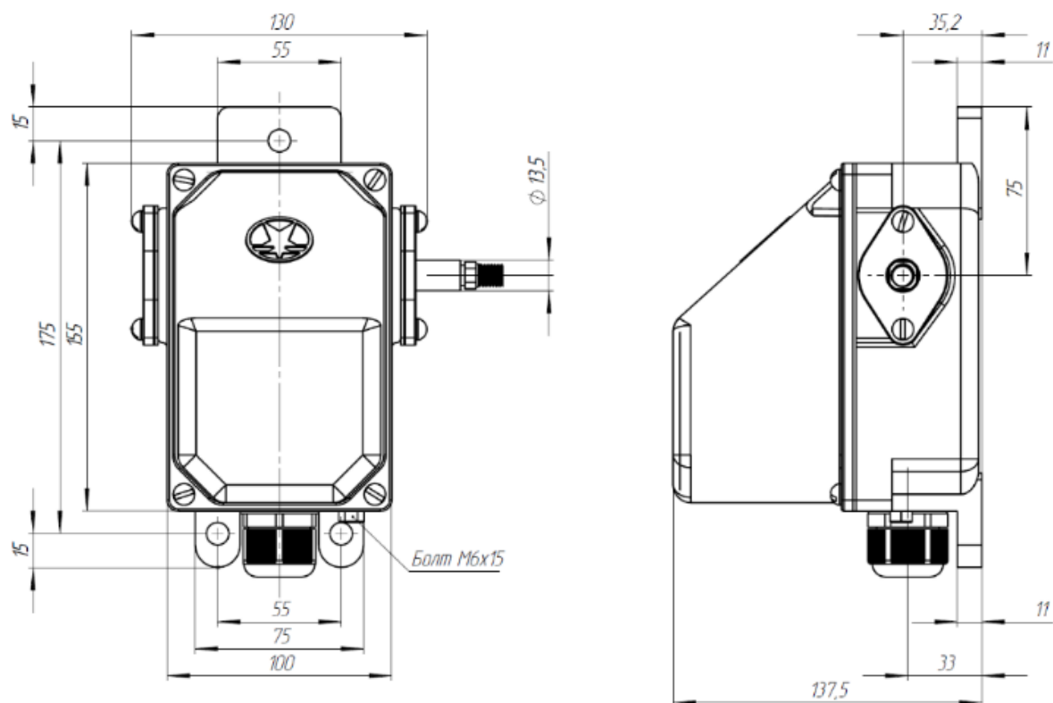
Габаритные размеры концевых выключателей
