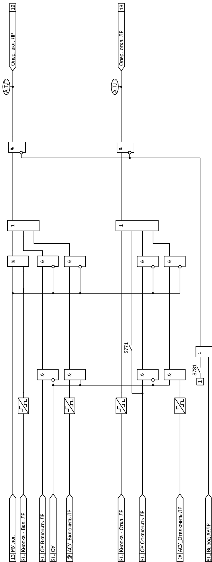
Рисунок Б.17 - Функциональная схема алгоритма формирования команд оперативного управления ЛР
