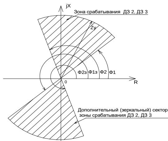
Рисунок 5 - Вид зон срабатывания ДЗ 2, ДЗ 3
