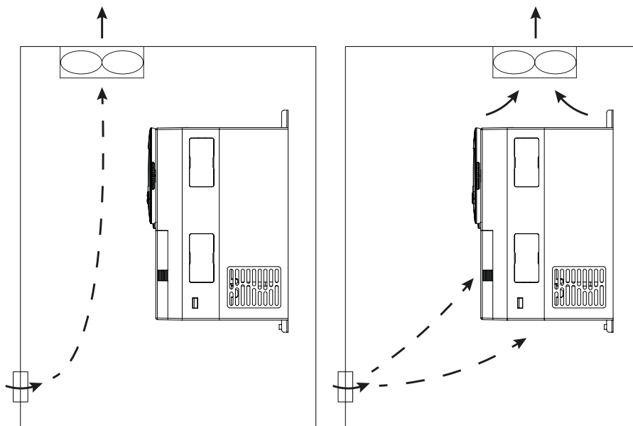
Некорректное размещение шкафового вентилятора
