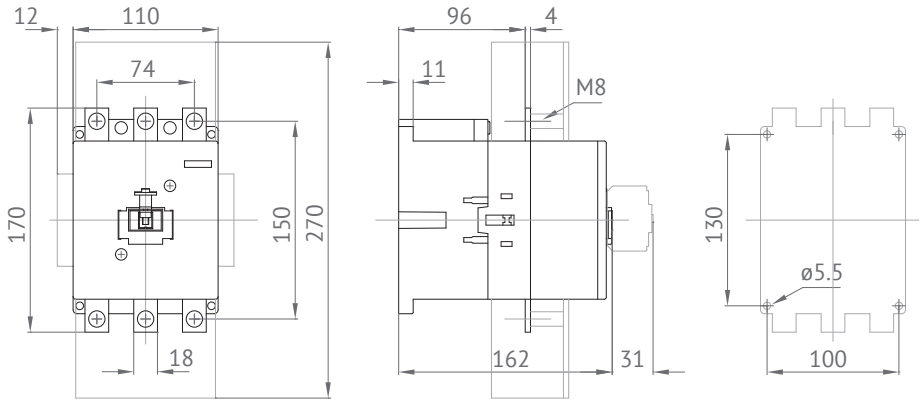
Контакты трехполюсные AC/DC
