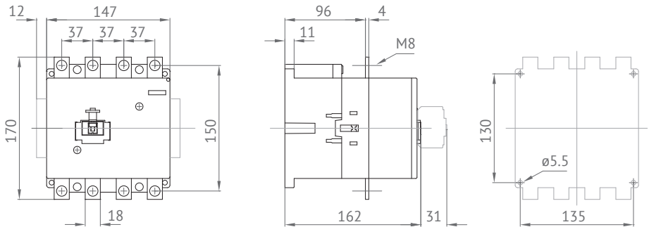
Контакты четырехполюсные AC
